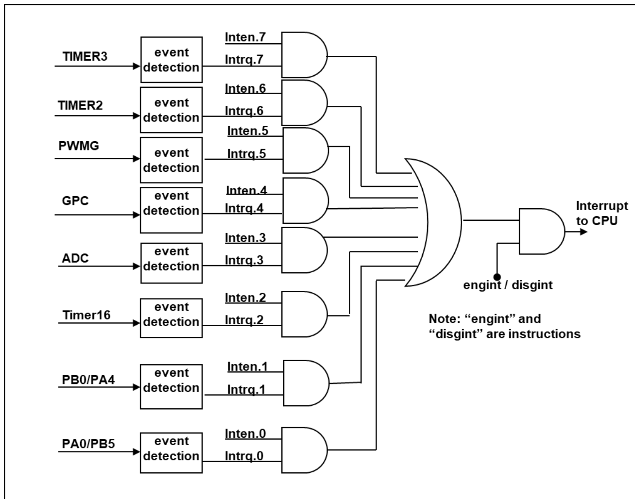
图 19：中断控制器硬件框图
