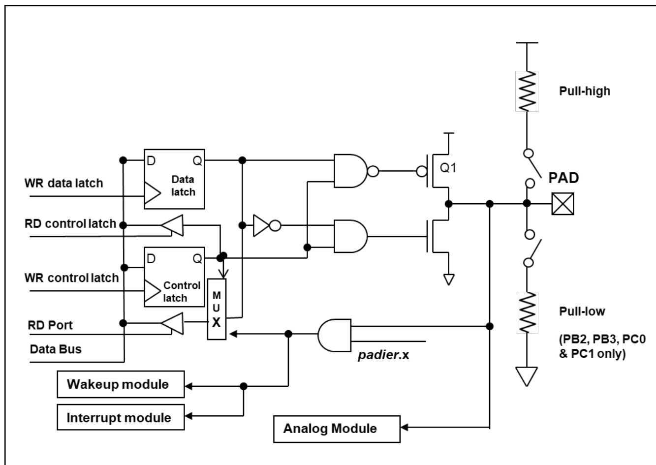
图 20: IO 引脚缓冲区硬件图
