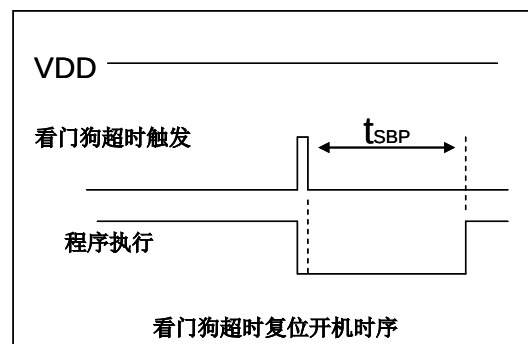
图 18：看门狗超时溢出时序图
