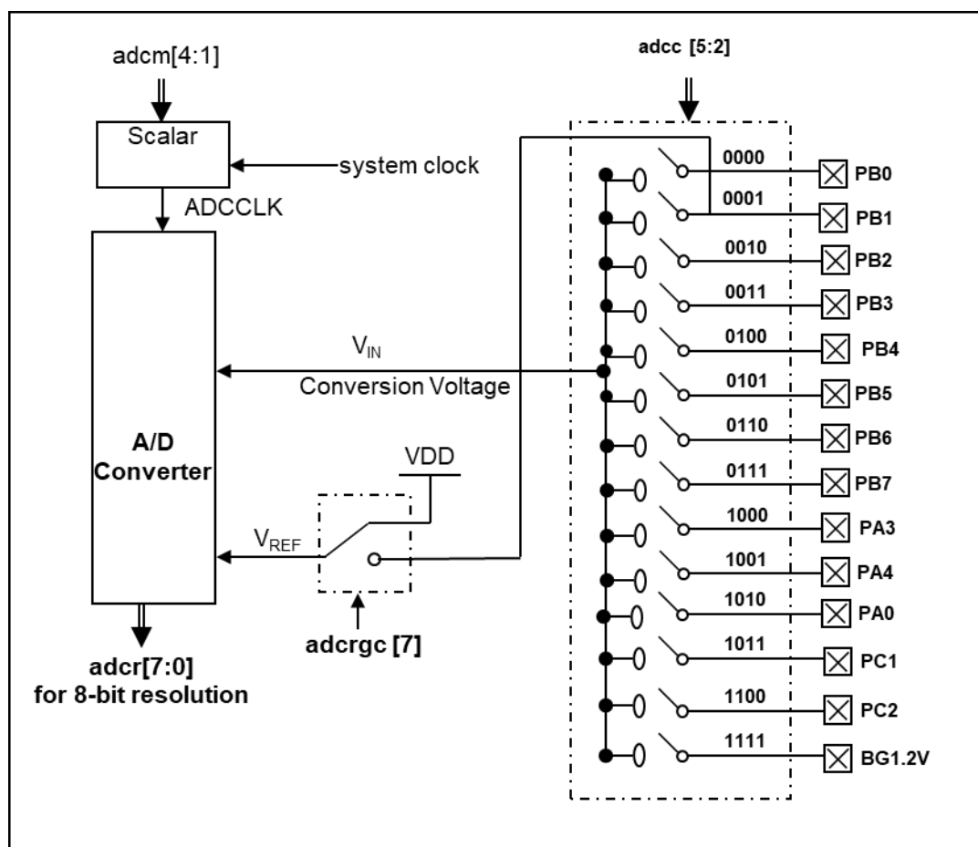
图 21: ADC 模块框图
