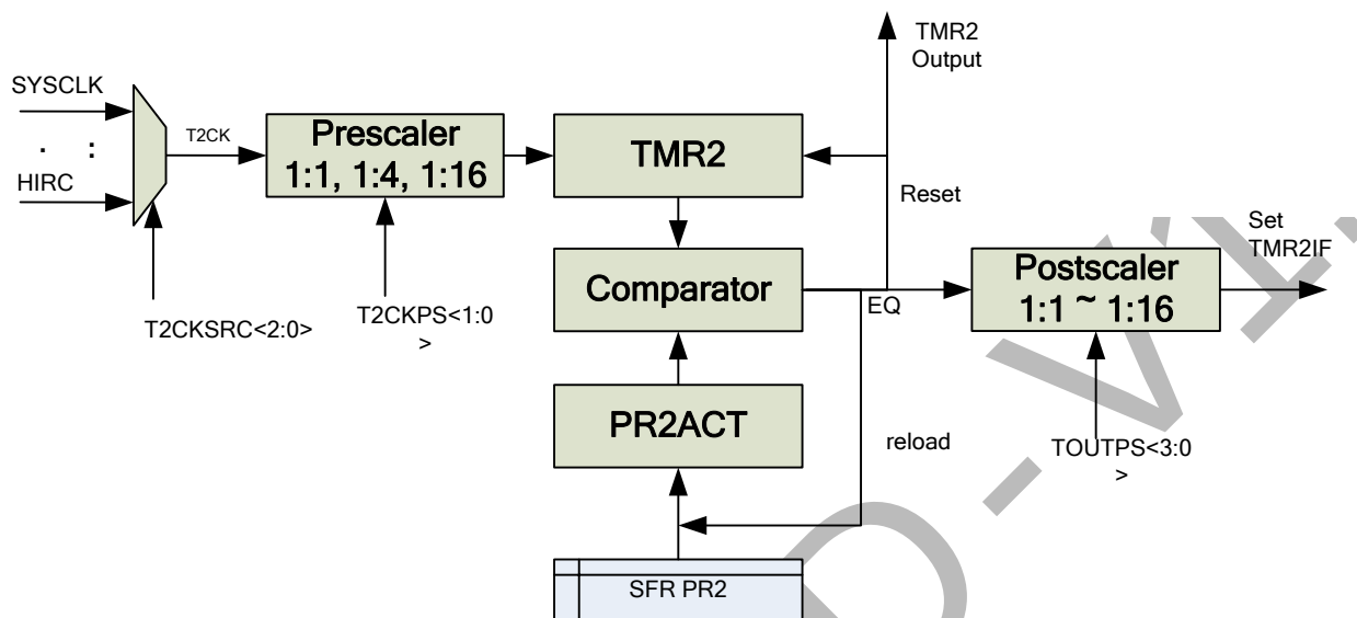
图 7.1 定时器 2 框图
