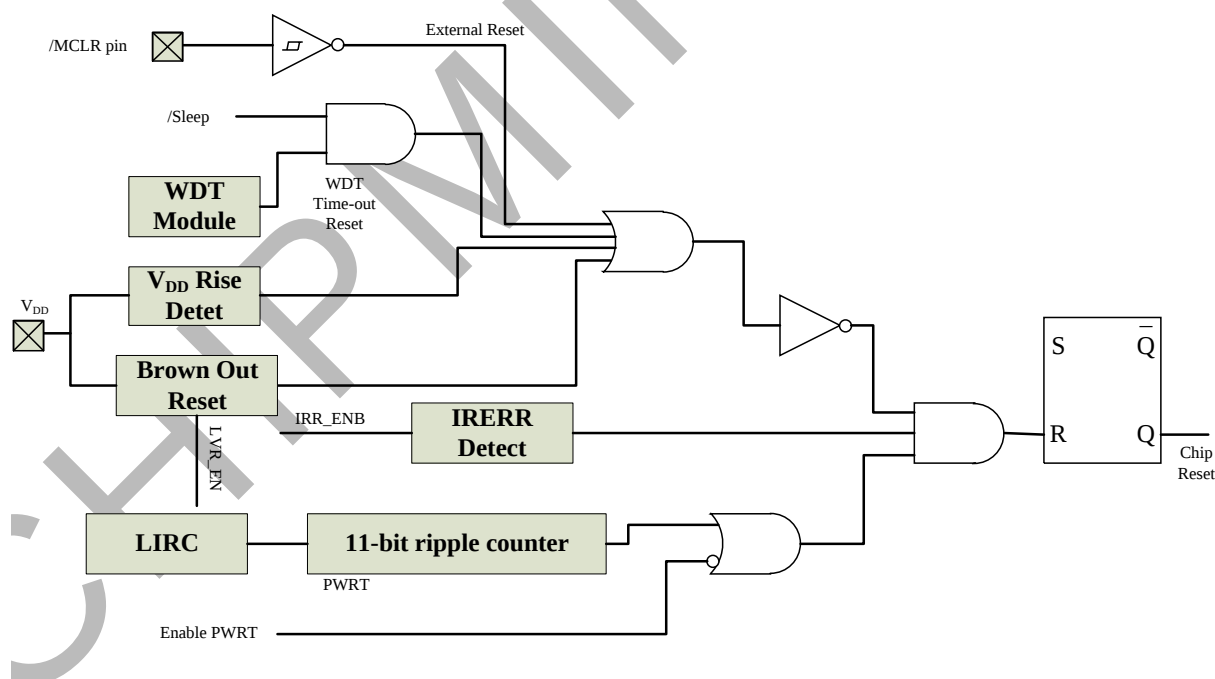
图 4.1 复位功能框图
