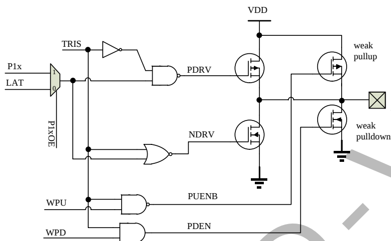
图 12.1 I/O 的一般结构
