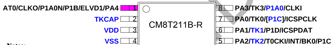
图 1.4 SOP8 脚位 A
