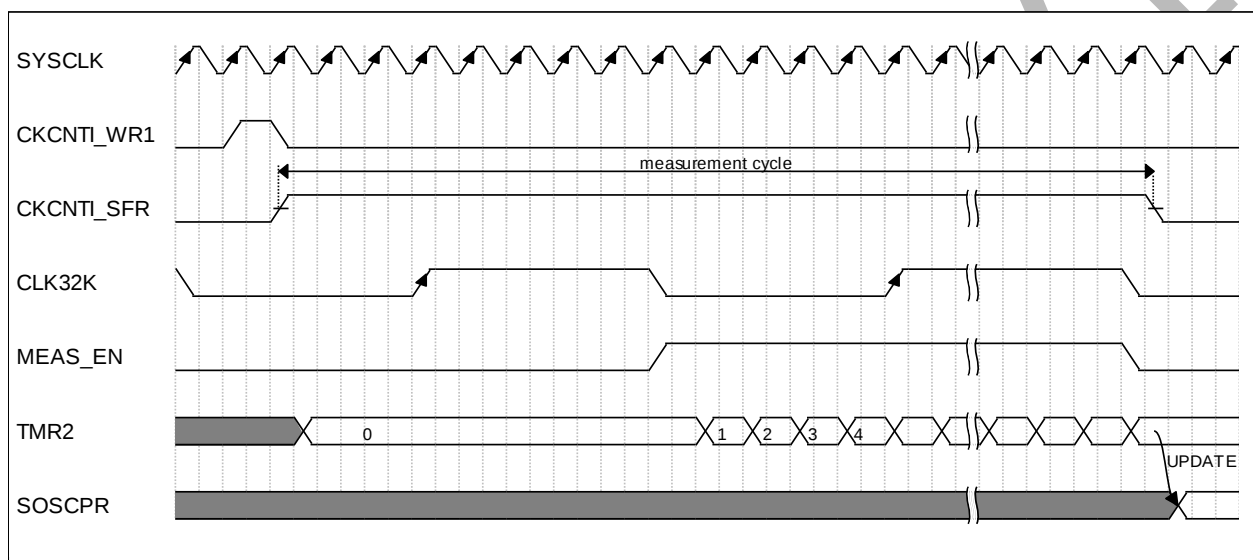
图 8.2 单次测量时序示意图（CLK32K 和 SYCLK 未按真实比例画）
