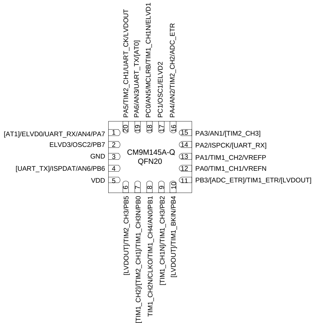
图 1.8 QFN20 脚位
