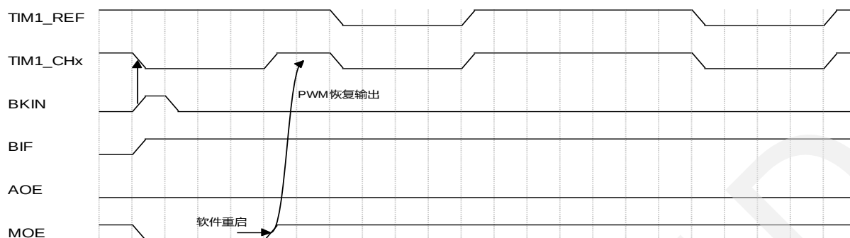
图 10.39 PWM 的软件重启
