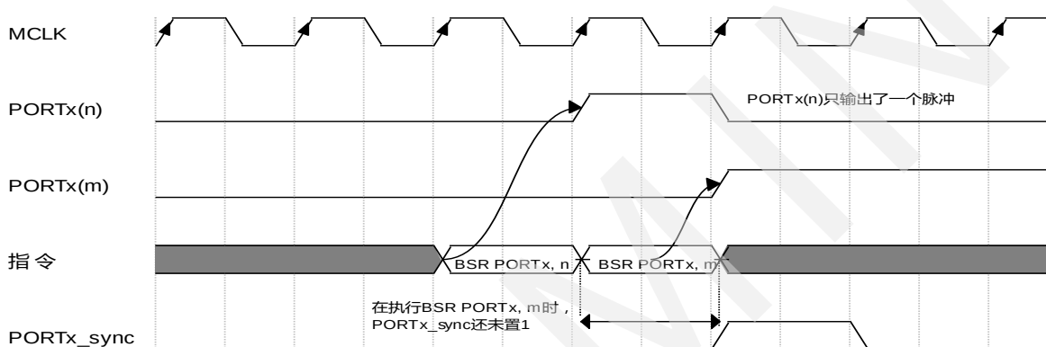
图 14.5 连续使用 RMW 指令对 PORTx 写操作的输出时序
