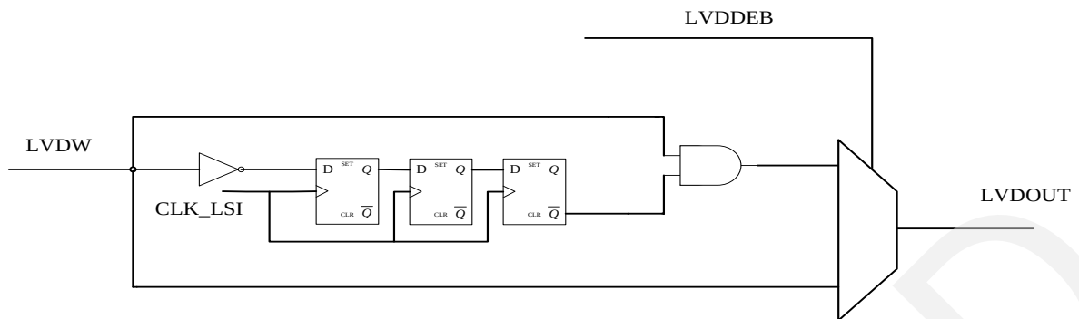
图 4.8.1 LVD 输出控制电路
