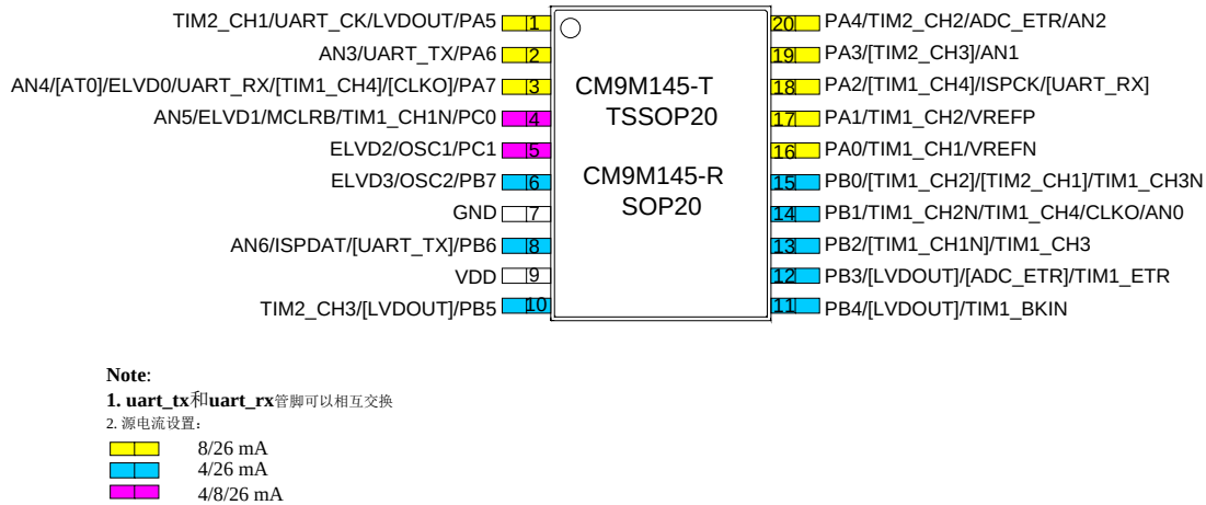
图 1.1 TSSOP20/ SOP20 脚位
