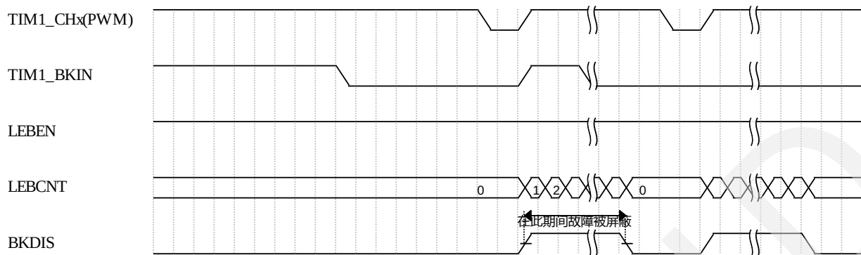
图 10.41 前沿消隐时序示意图
