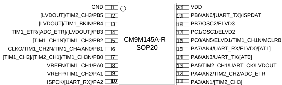
图 1.2 SOP20 脚位
