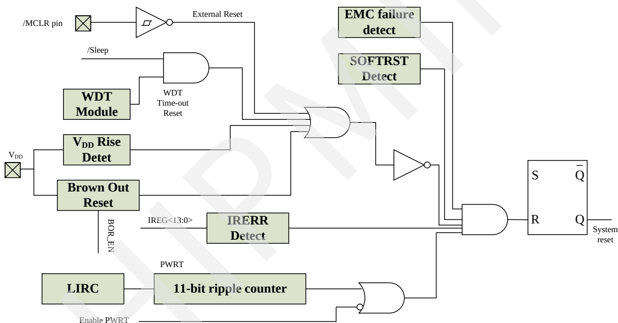
图 4.1 复位框图
