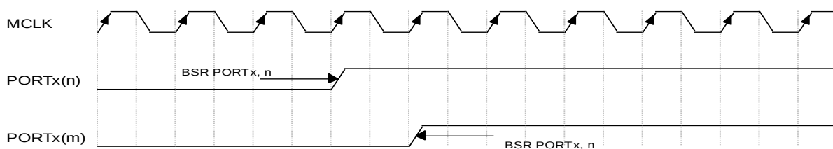
图 14.4 连续使用 RMW 指令对 PORTx 写操作的期望时序
