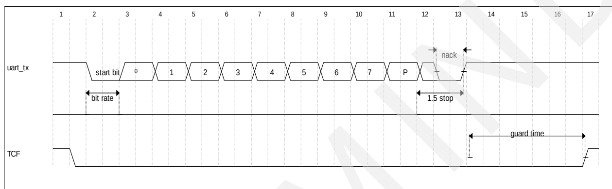
图 13.7 智能卡模式时序图
