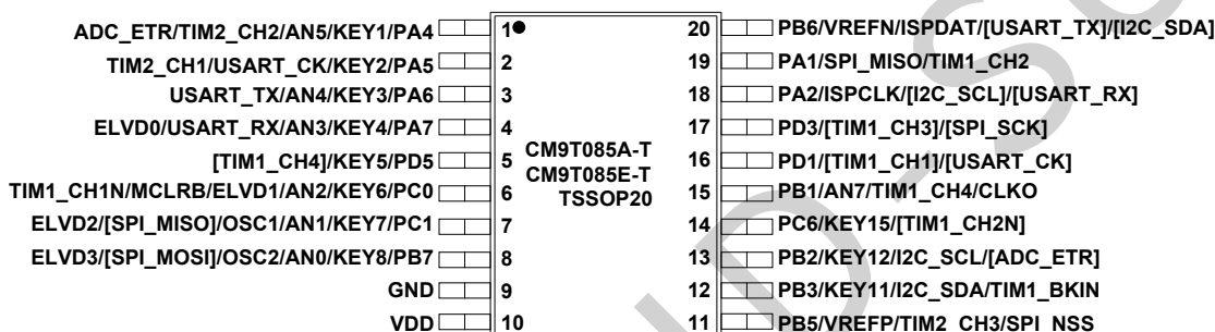
图 1-3 TSSOP20
