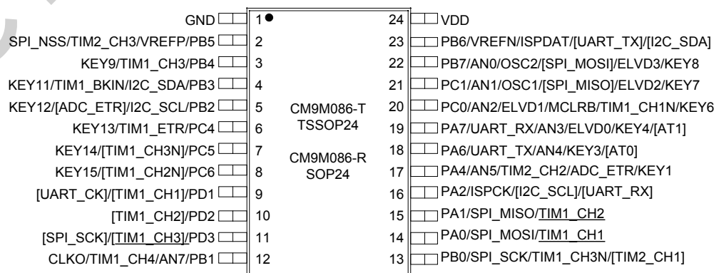
图 1.3 SOP24/TSSOP24 脚位
