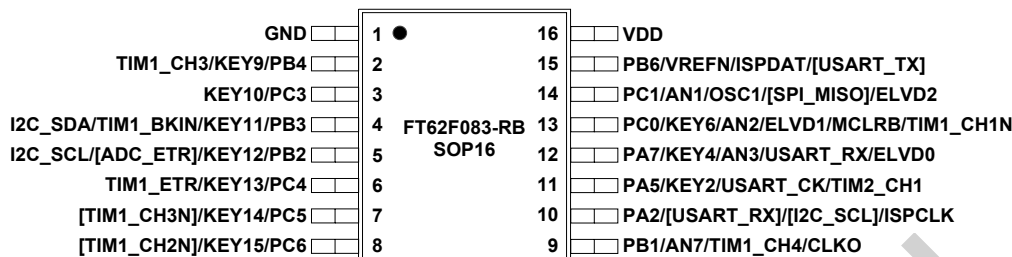
图 1-2 SOP16
