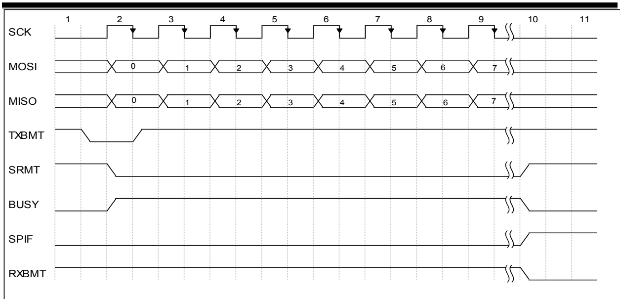
图 13.5 数据处理时序图
