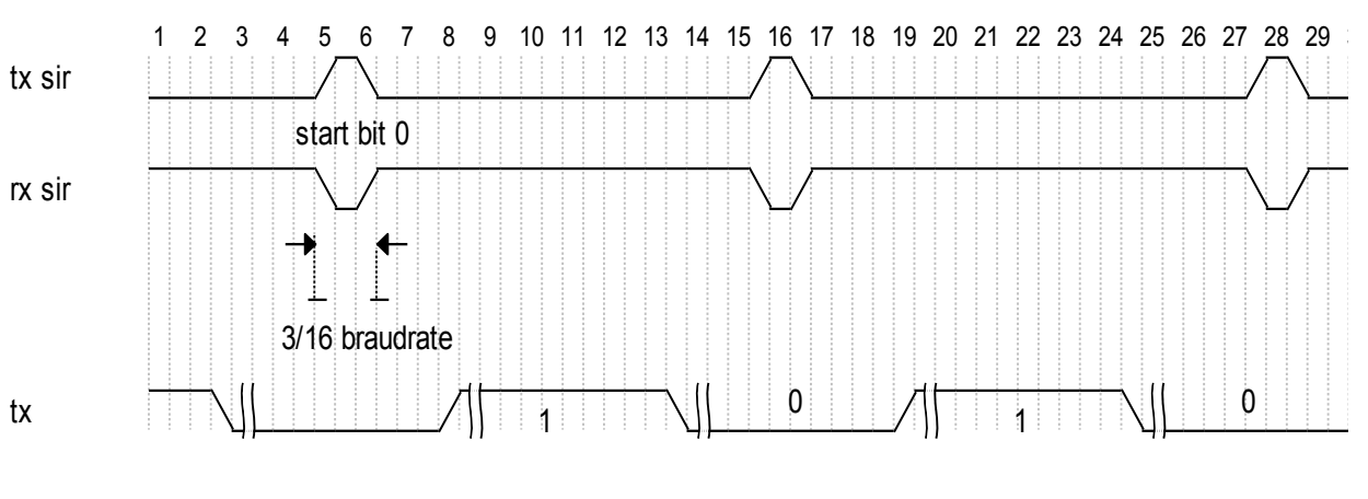
图 15.5 红外模式时序图
