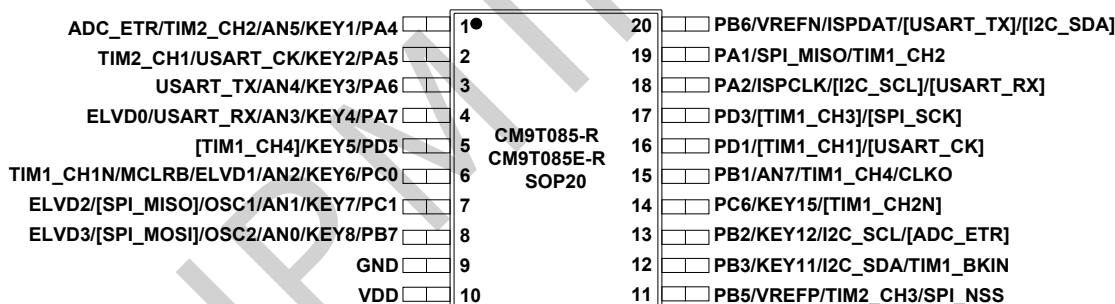
图 1-4 SOP20
