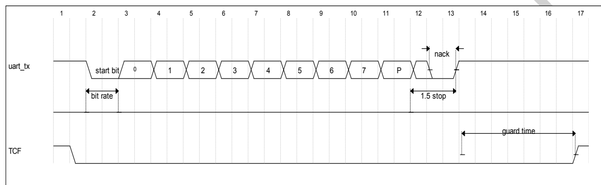
图 15.7 智能卡模式时序图
