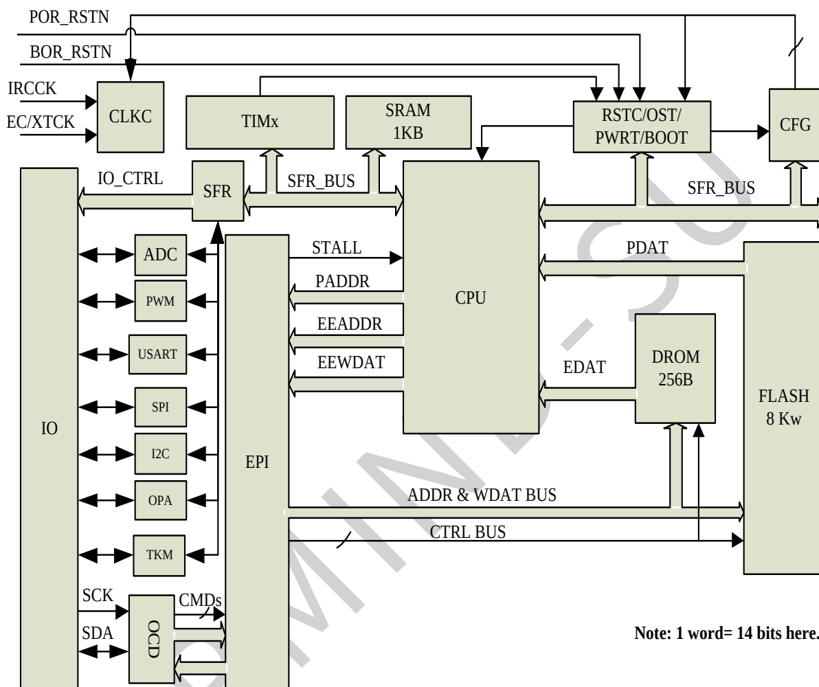
图 1.1 芯片整体功能框图
