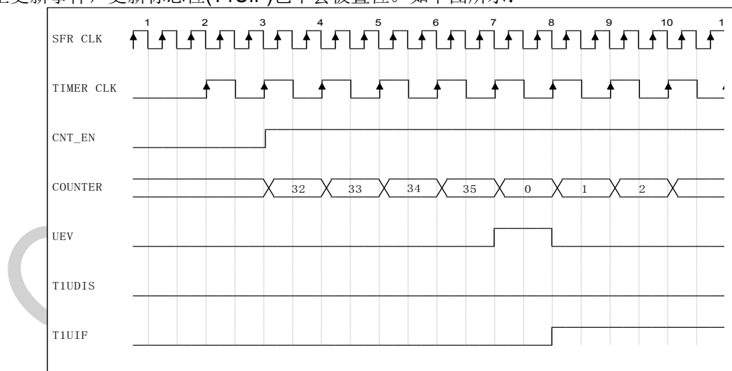
图 10.8 更新事件下且 T1UDIS=0 ，更新标志位变化图
