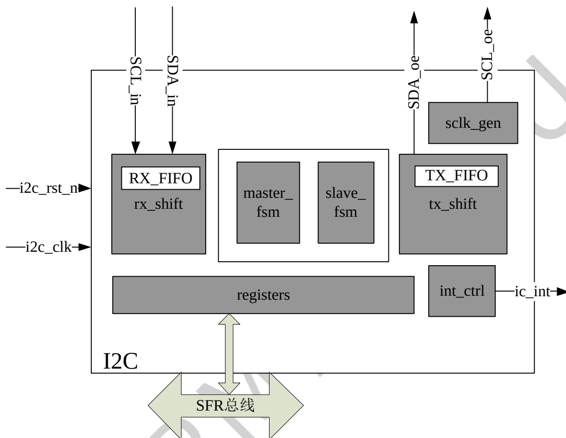
图 14.1 I2C 原理框图
