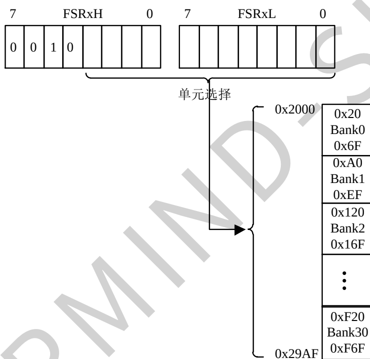
图 3.6 线性数据存储器映射
