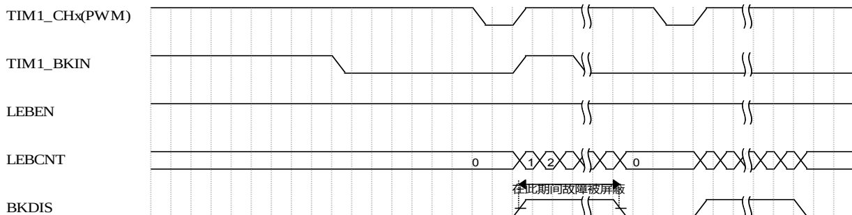
图 10.37 前沿消隐时序示意图
