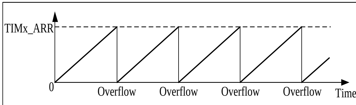
图 11.3 向上计数器
