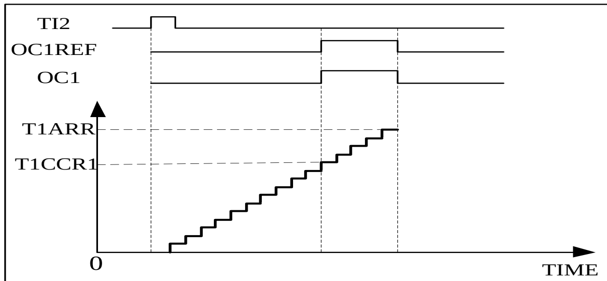
图 10.29 单次脉冲应用示意图
