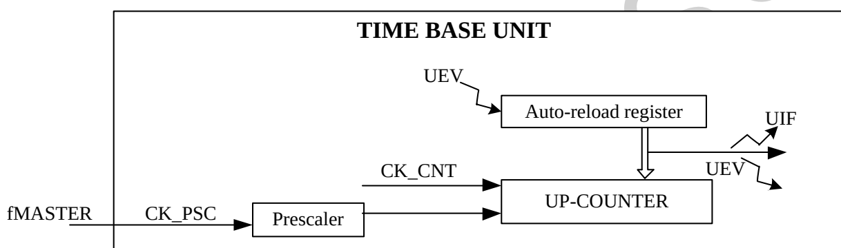
图 12.1 TIM4 原理框图
