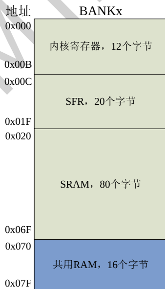
图 3.1 存储区构成
